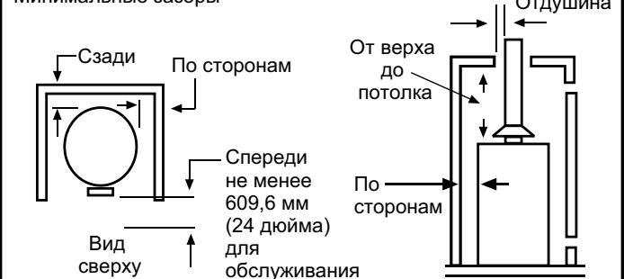
Рисунок 2 Минимальные зазоры
