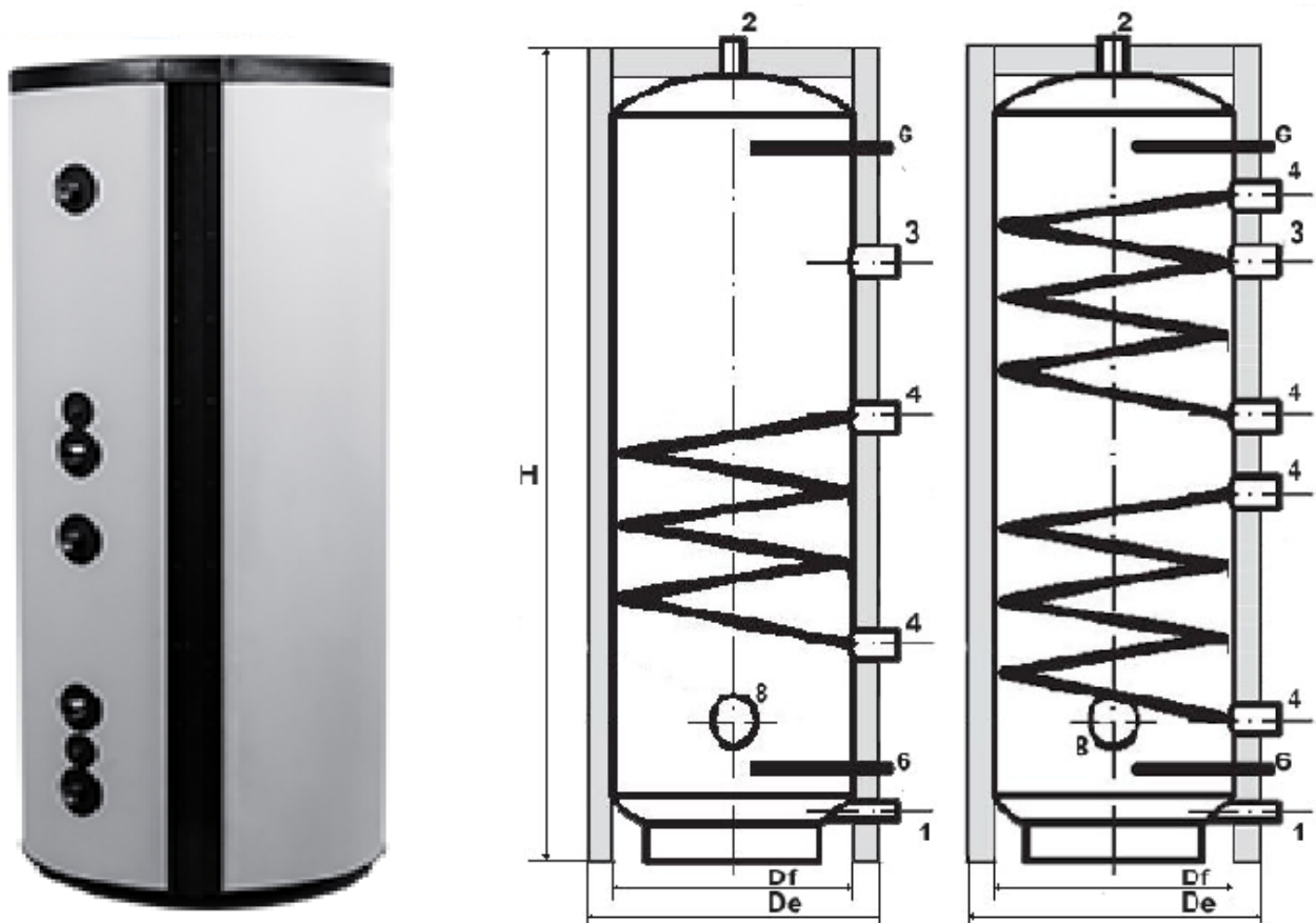
Рис. 1 Подключения и технические характеристики
